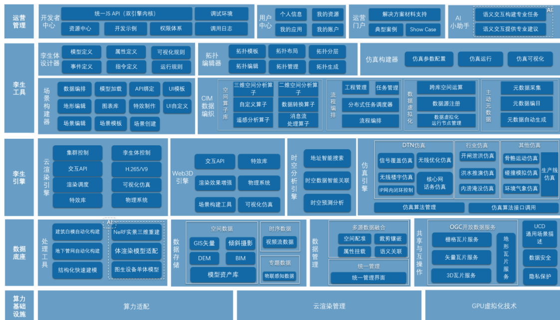
图4-1 数字孪生平台产品功能架构
